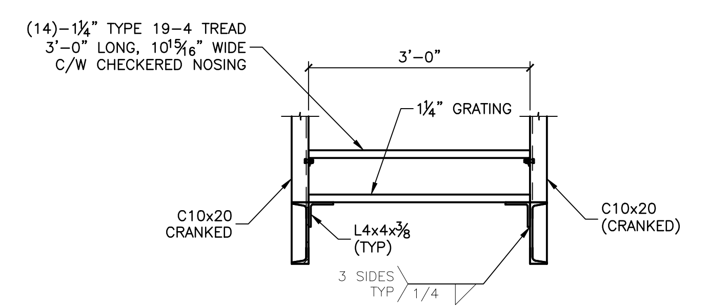
SECTION E SCALE: 3/4" = 1'-0"
