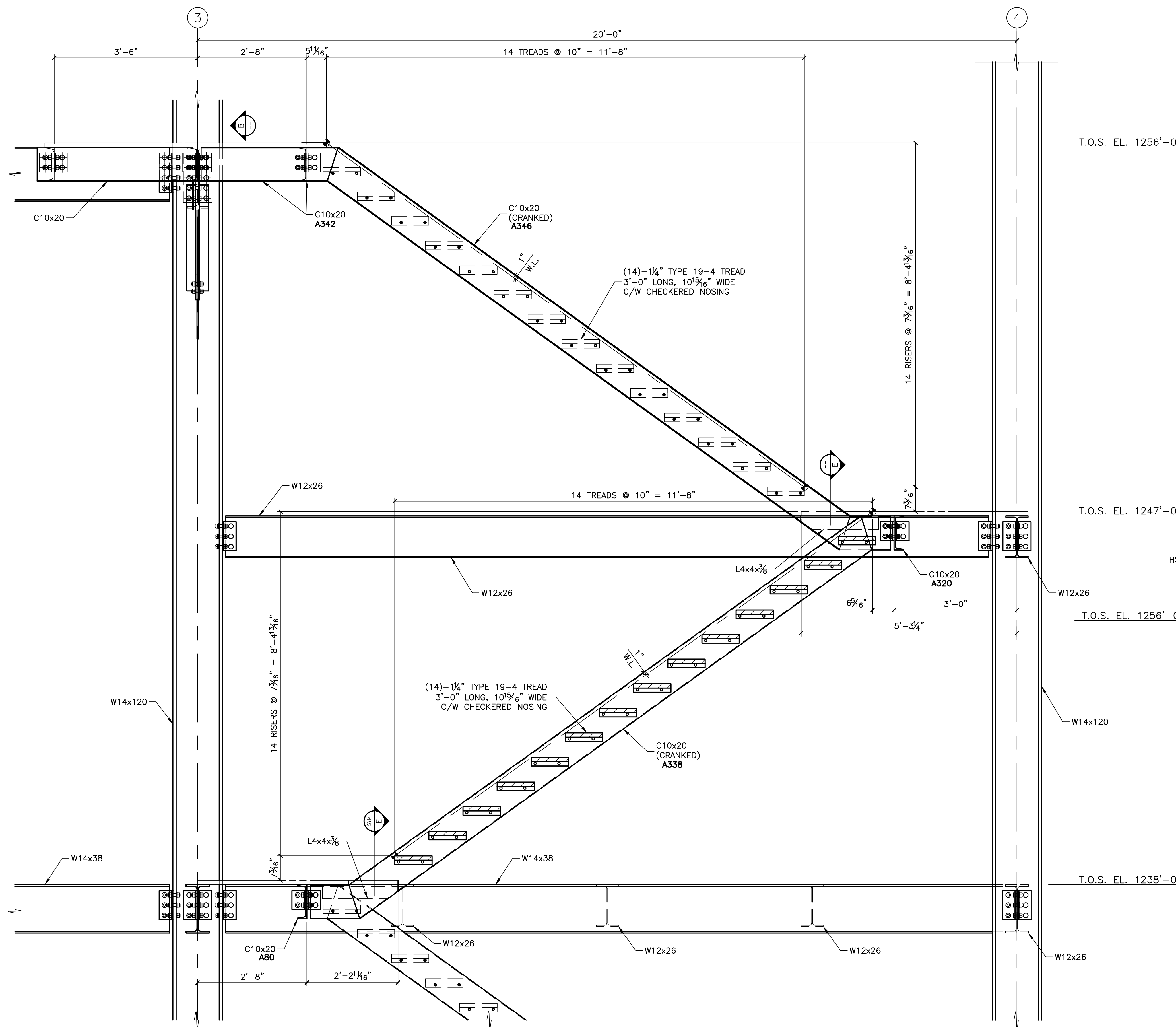
SECTION A SCALE: 3/4" = 1'-0"
